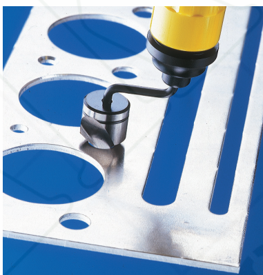
POGŁĘBIACZ "GT-U" GRAT-TEC RotoDrive EL6500GT
