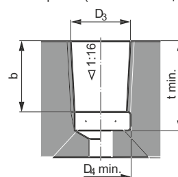
Рекомендуемая подготовка глухих отверстий (минимальная длина)
