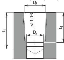
Цилиндрическое сверление и подготовка конического отверстия расширителем
