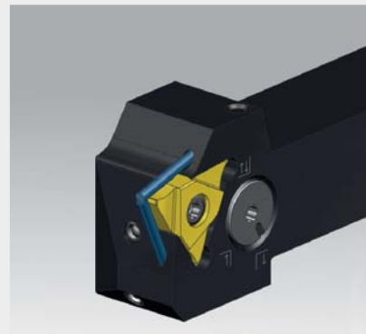
Kühlmittelzufuhr auf Span- und Freifläche
