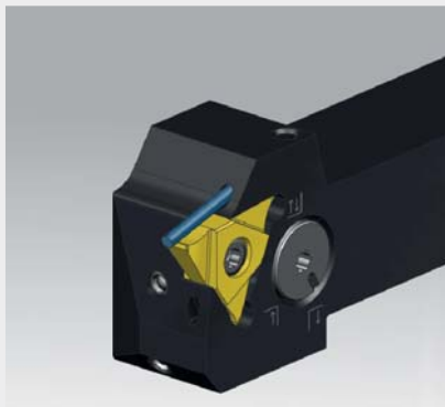
Kühlmittelzufuhr auf die Spanfläche
